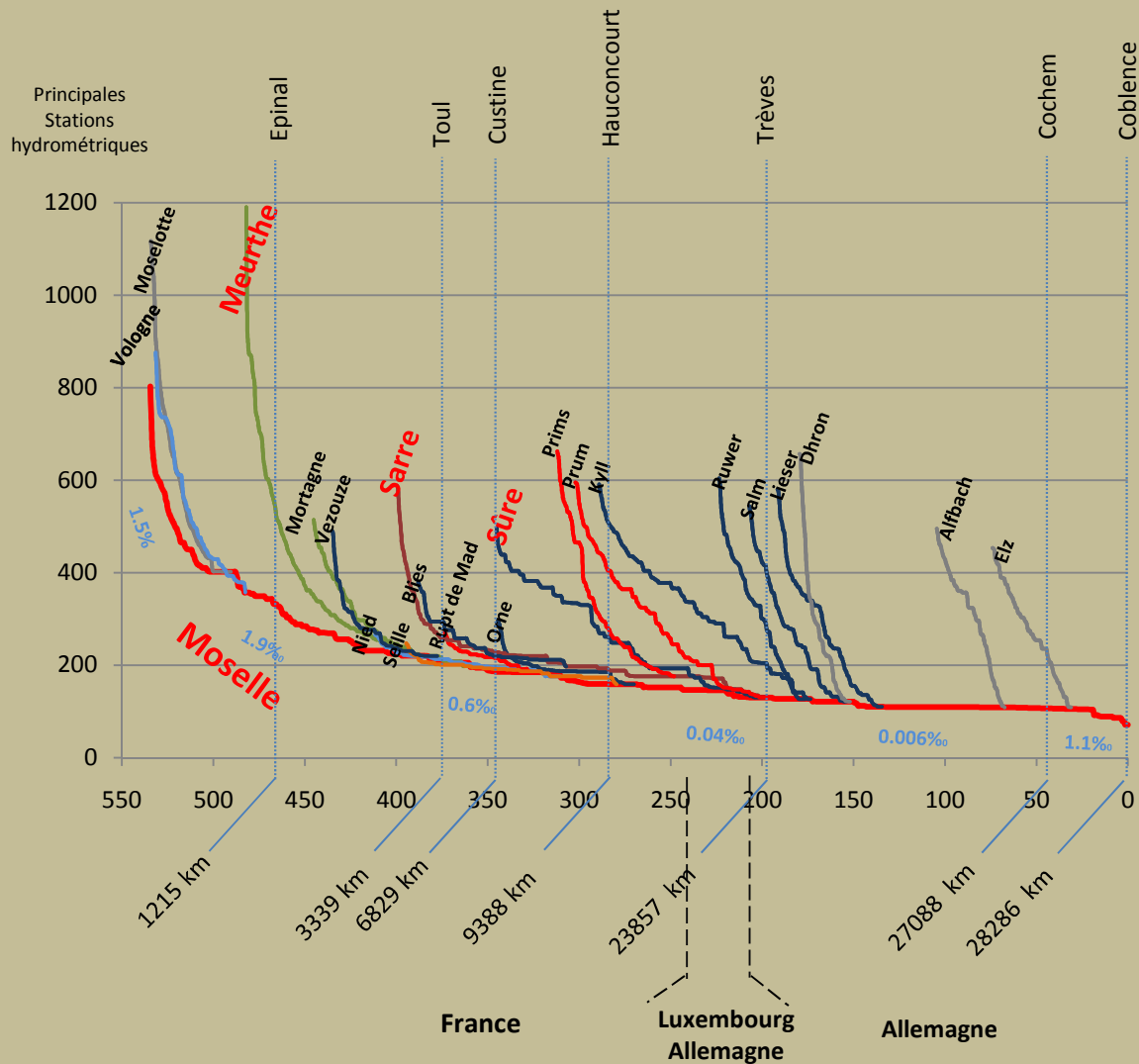
Profil en long de la Moselle et affluents
