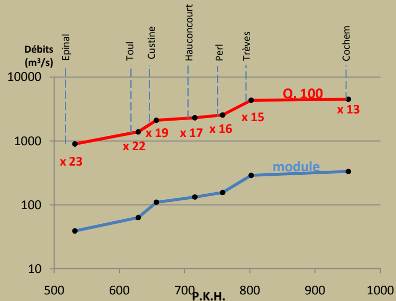
Profil des Q.100 et modules
