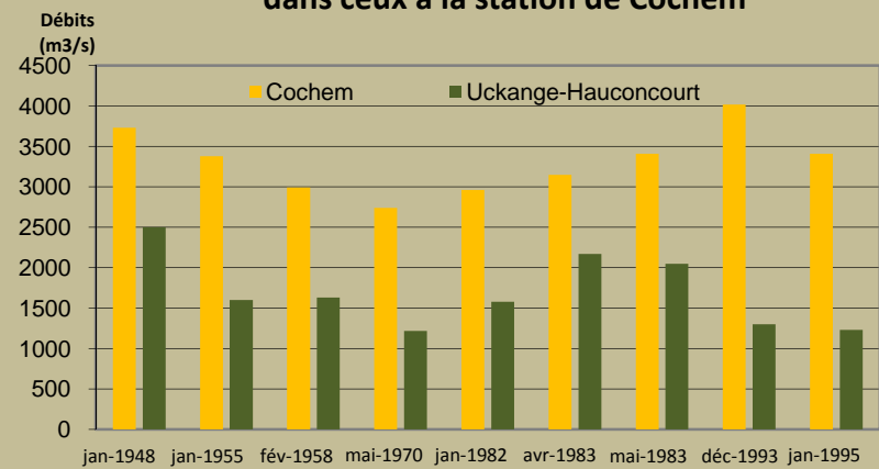
Part des débits à la station de Uckange dans ceux à la station de Cochem
