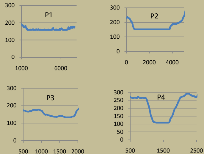
Profils en travers dans la vallée de la Moselle
