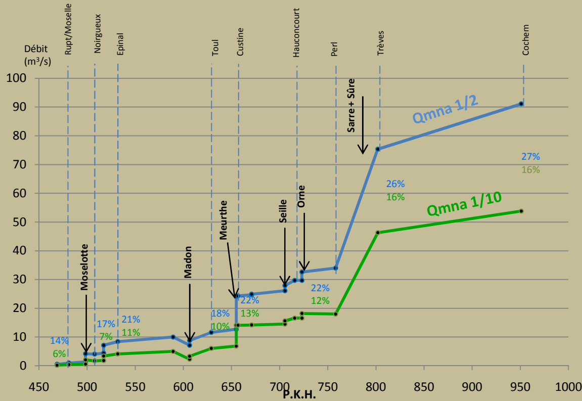
Profil hydrologique de la Moselle: débits mensuels d'étiage de fréquence 1/2 et 1/10
