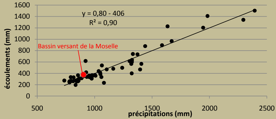
Relation précipitations/écoulements sur la bassin de la Moselle
