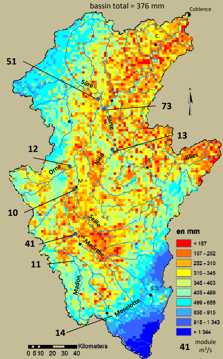
Lame d'eau écoulee et modules
